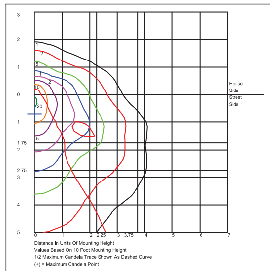
D-175w-MH-MWP
